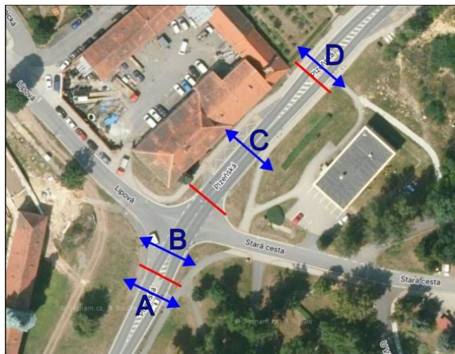
Intenzita chodců přecházejících v jednotlivých úsecích silnice I/27
